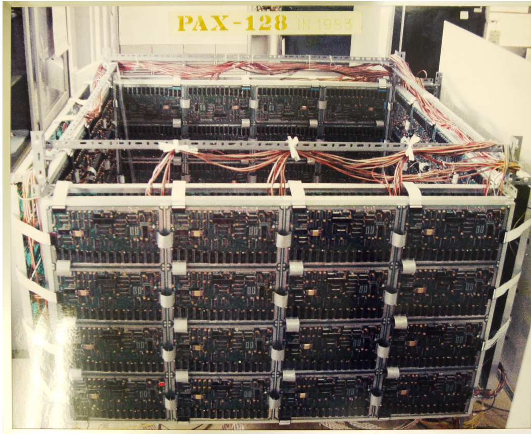
PAX-128 4Mflops。 筑波大学、星野ら
